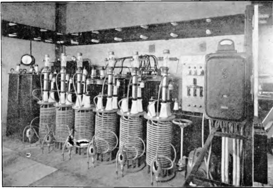
Batterij gelijkrichters 3e trap P. C. L. L.
